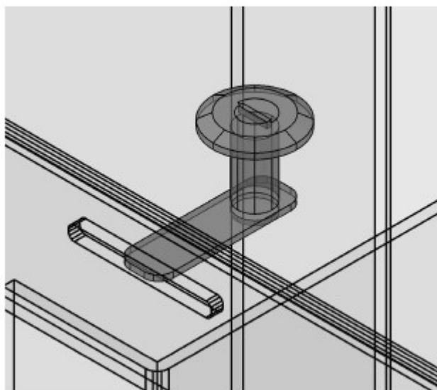
Rysunek 4. Zamek zamontowany w pokrywie, ryglowany w otworze wykonanym w obudowie kosza
