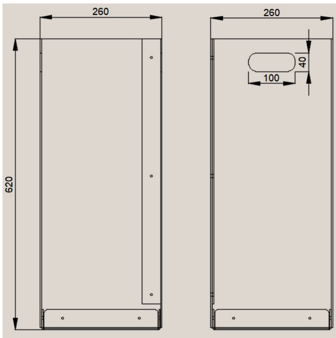
Rysunek 6. Widok rzutów wkładu wraz z wymiarami
