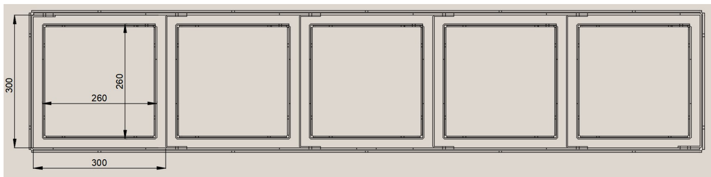
Rysunek 1. Widok z góry na kosz bez pokrywy. W środku podane wymiary wewnętrzne jednej komory i zewnętrzne wkładu
